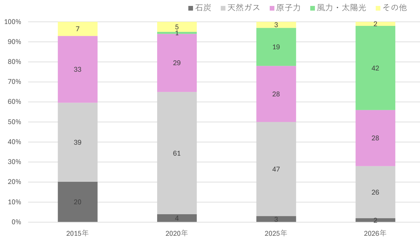
図2 バージニア州の電源構成計画
