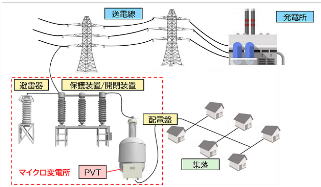
図 マイクロ変電所による電力供給イメージ
