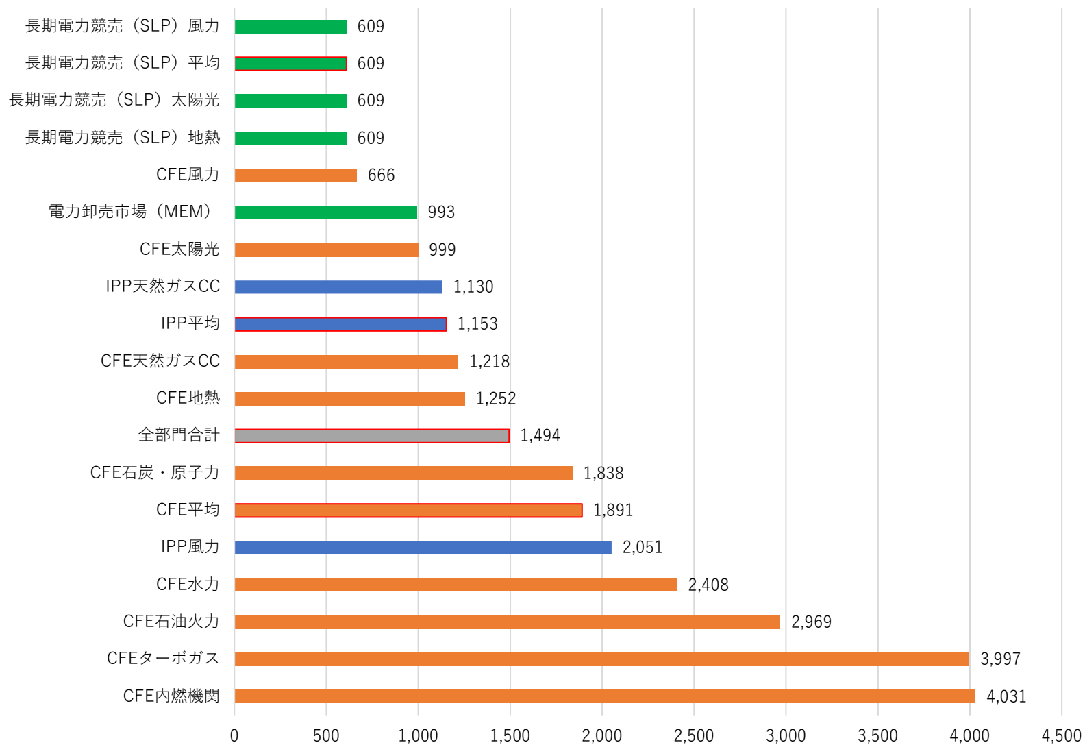
図 CFE SBの調達部門・発電技術別電力調達コスト（ペソ/MWh） （2023年3月）
