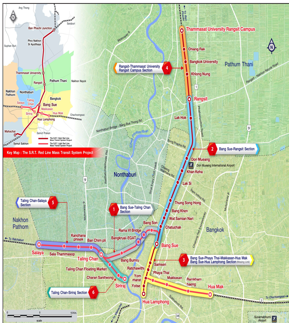
図 レッドライン事業路線計画図(タイ国有鉄道提供)
