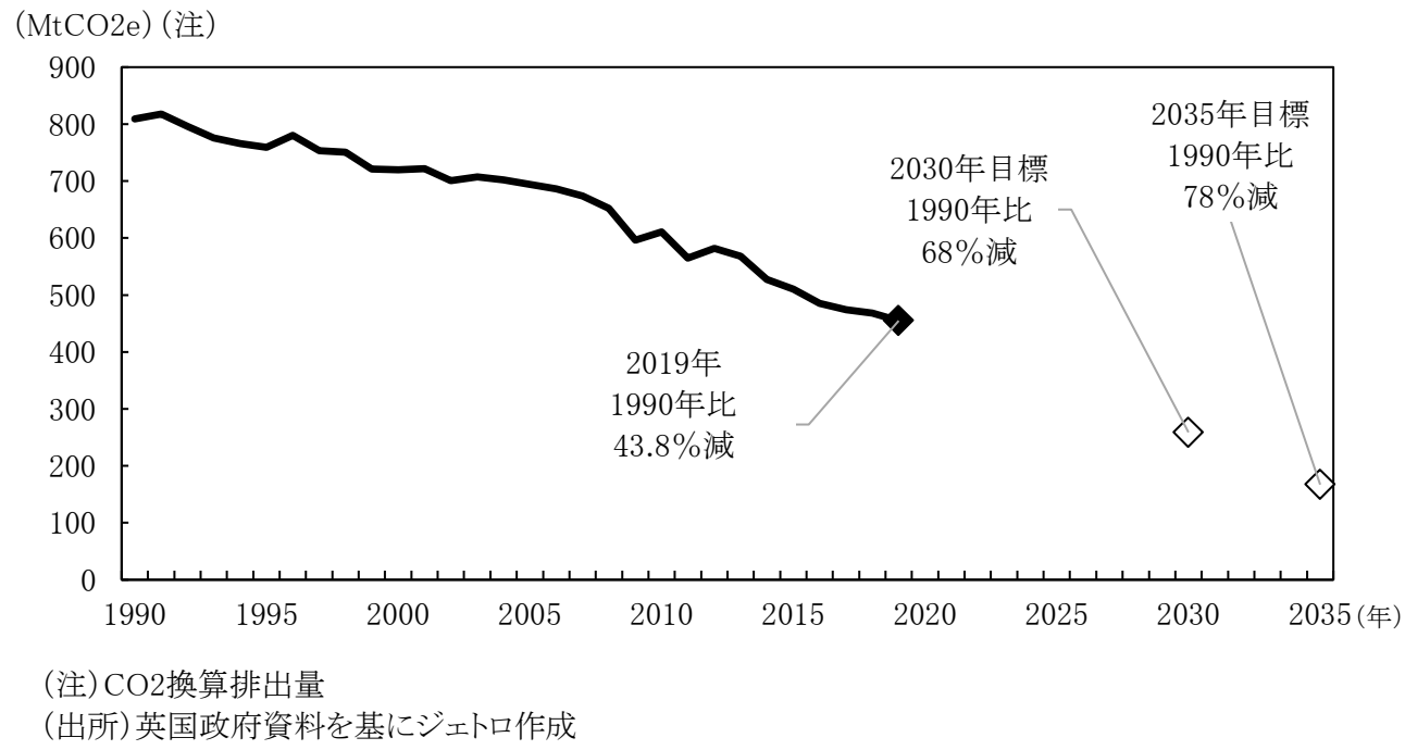
図1 英国の温室効果ガス(GHG)排出量の推移
