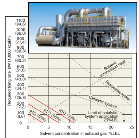
Regenerative Thermal Oxidizer(RTO)
