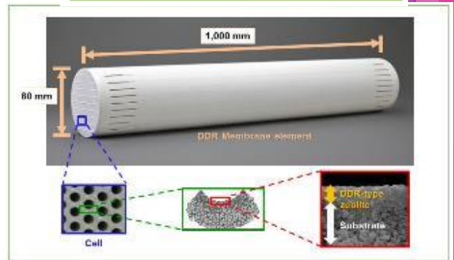
DDR 膜パイプライン
