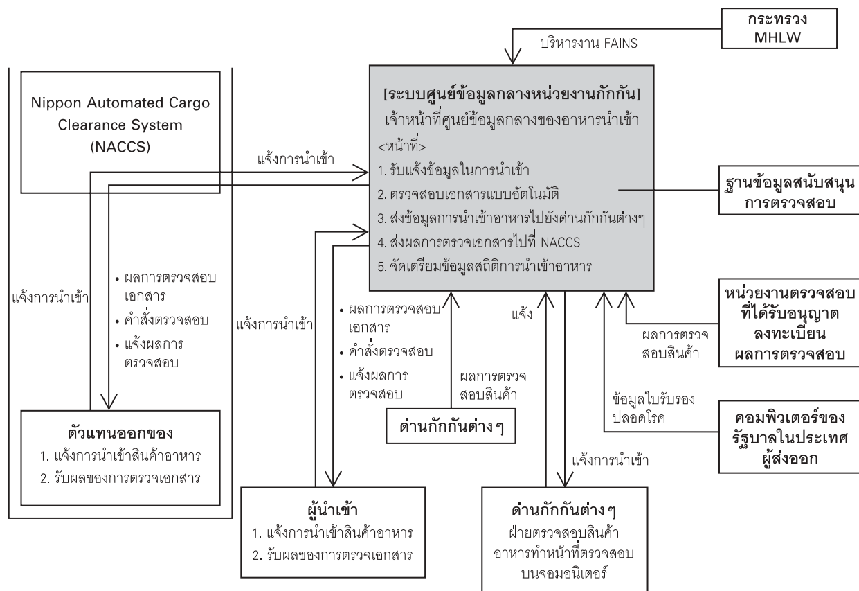
ภาพที่ 9 ระบบสนับสนุนการกำกับดูแลสินค้าอาหารนำเข้าด้วยคอมพิวเตอร์ (FAINS)
