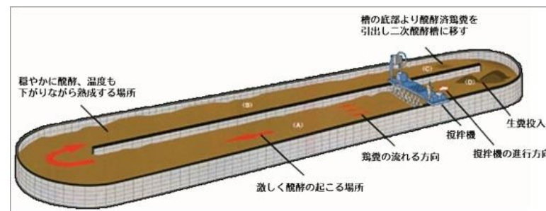
鶏糞発酵システム
