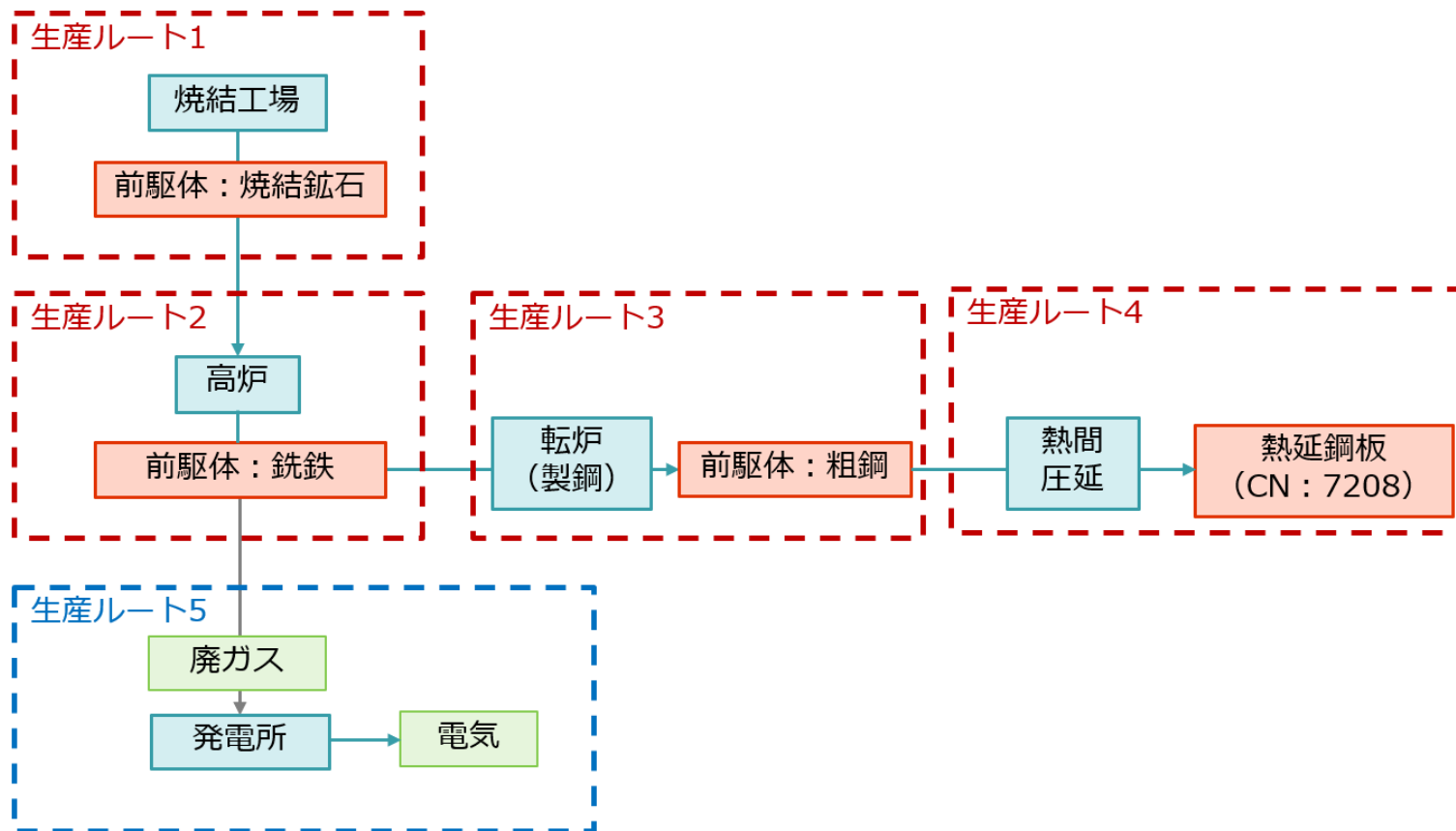
図3：熱延鋼板の製造工程の例（高炉の場合）
