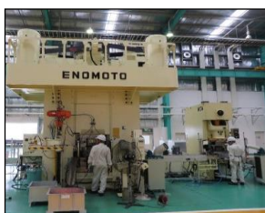
熱間鍛造ライン(一部)
